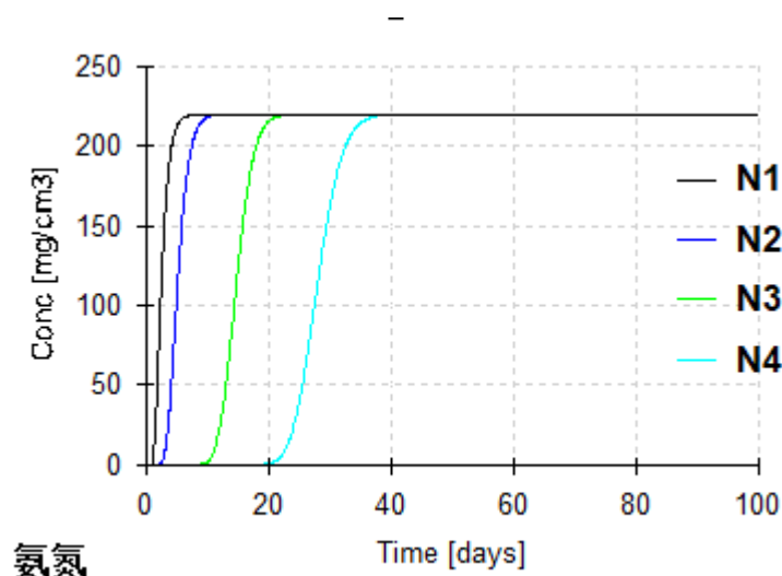
图4-7 土壤环境中NH 3 -N预测浓度图
